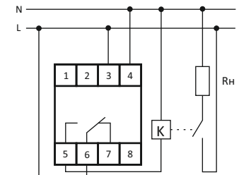
Rn - подключаемая нагрузка
