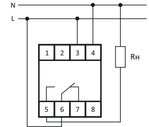
Rn - подключаемая нагрузка
